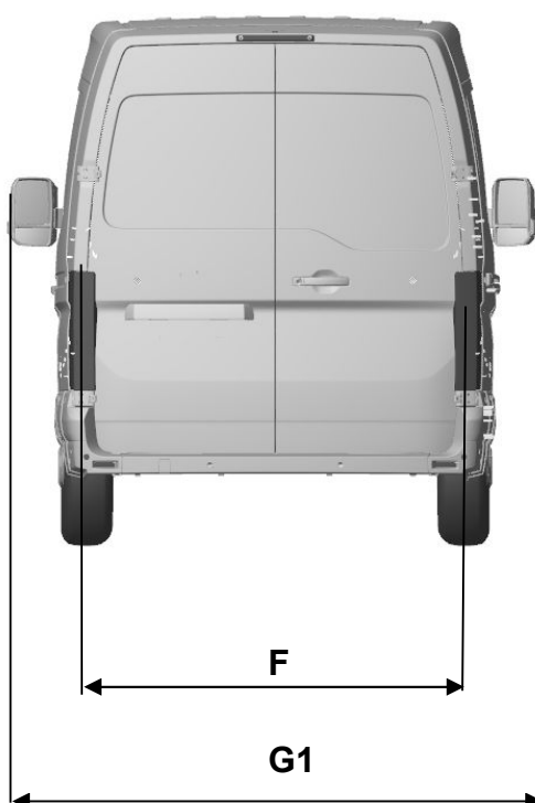
VISTA DE TRÁS
